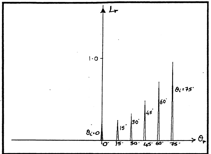
(d) \sigma_h = 0.001 , T = 0.01 , \lambda = 0.01
