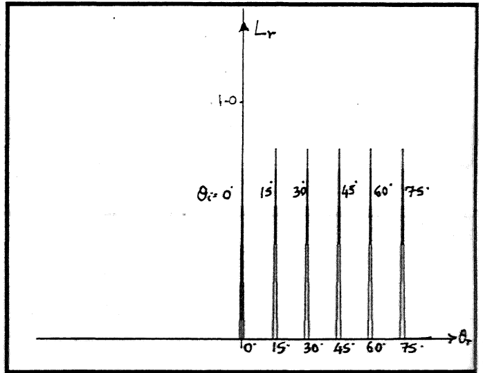
(d) \sigma_h = 0.001 , T = 0.006 , \lambda = 0.5
